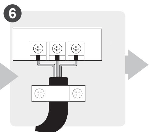
6 Conectare Cablaj (nu este aplicabil pentru unele locații din America de Nord)
