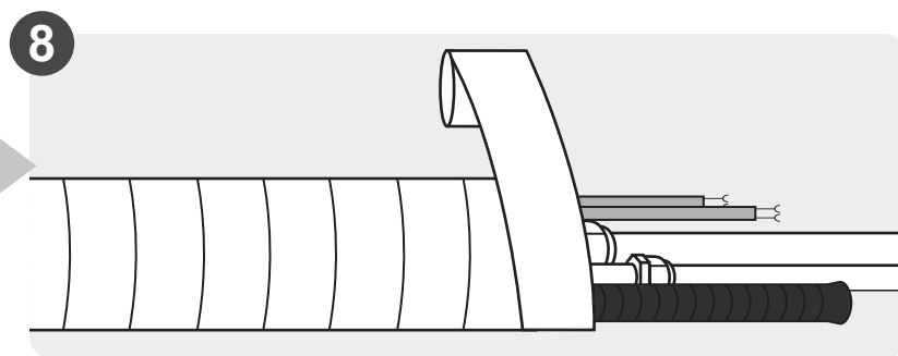
8 Îvelire Conducte Și Cablu (nu este aplicabil pentru unele locații din America de Nord)
